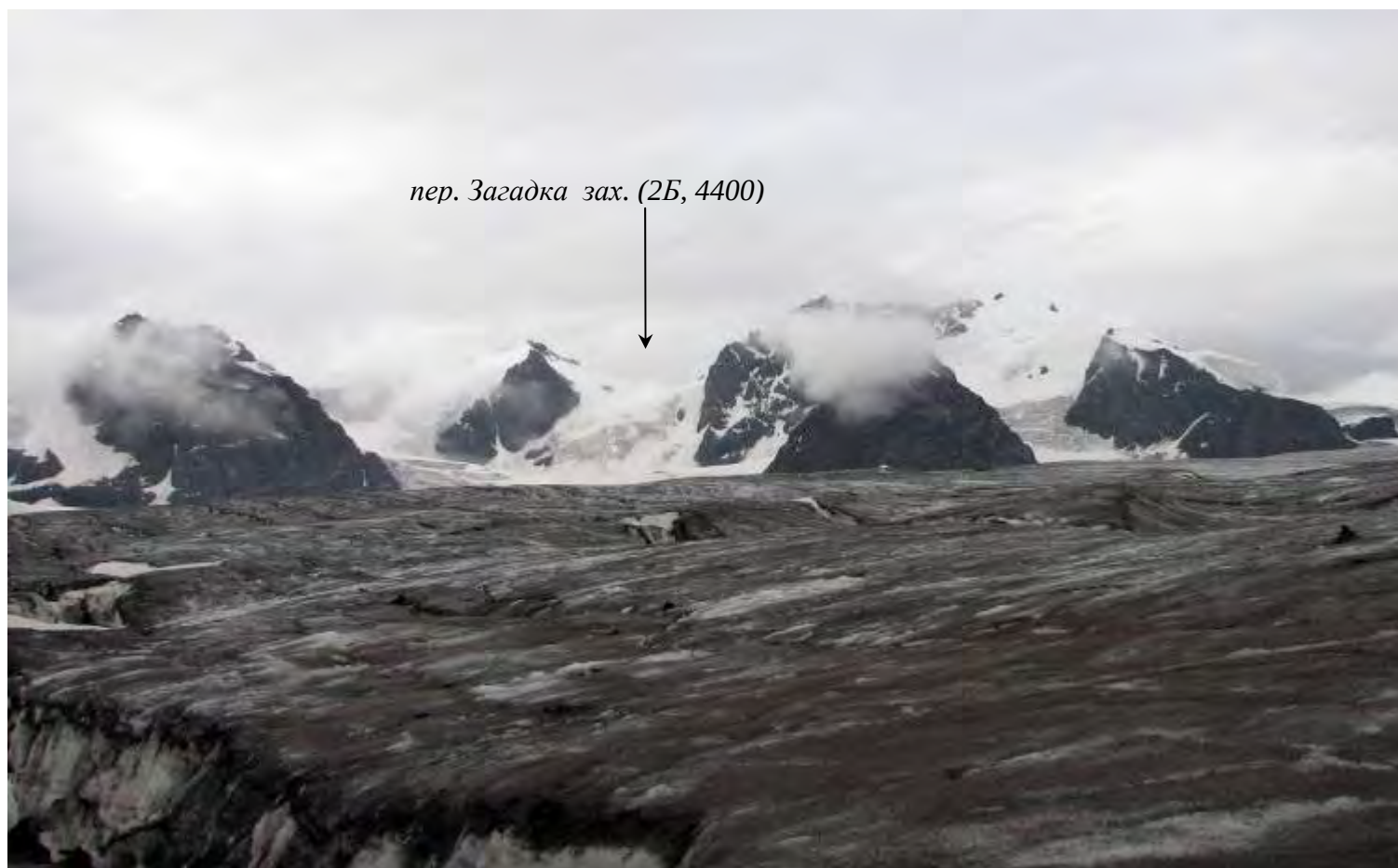
Фото 102. Льодовик Колпаковського.
