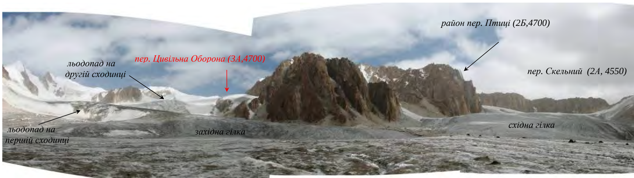
Фото 30. Льодовик Віялоподібний.
